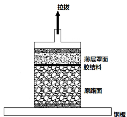
图1 拉拔试验原理。
